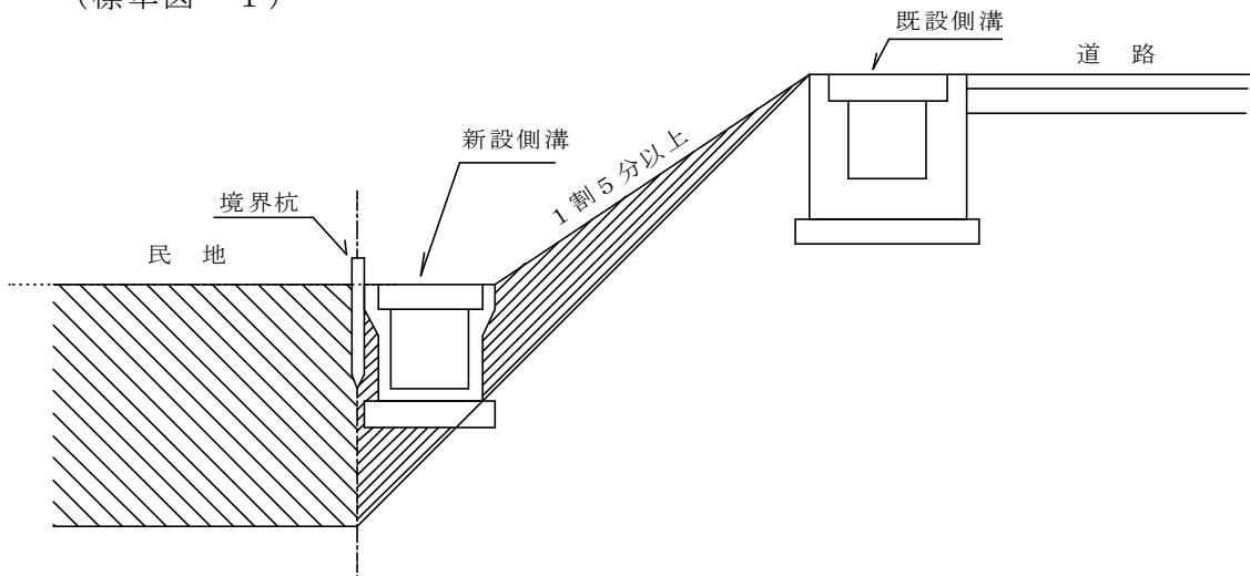
(標準図－２)
