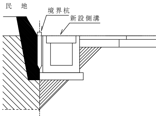
(標準図－５)
