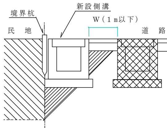
(標準図－２)
