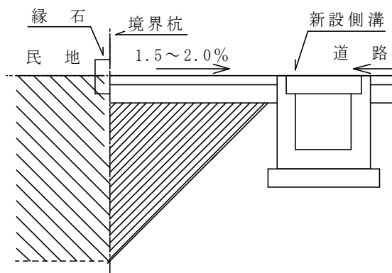
(標準図－３)
