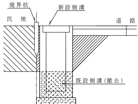
(標準図－４)
