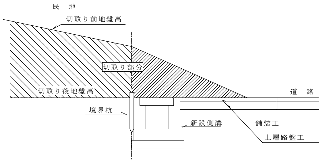
(標準図－1)
