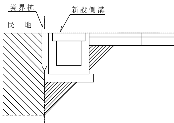
(標準図－５)
