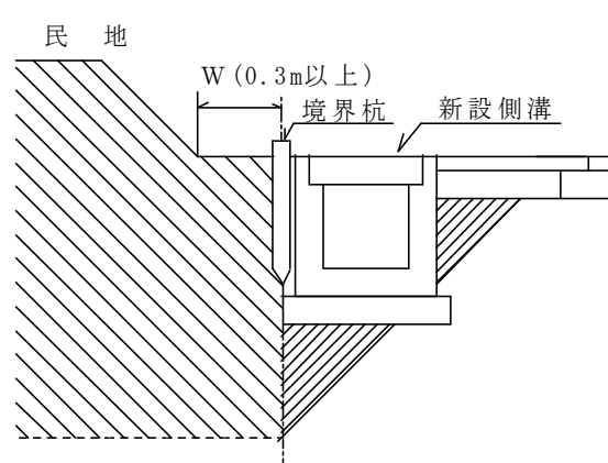
(標準図－６)
