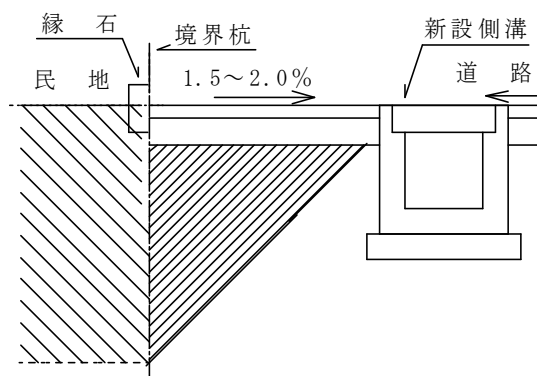
(標準図－３)
