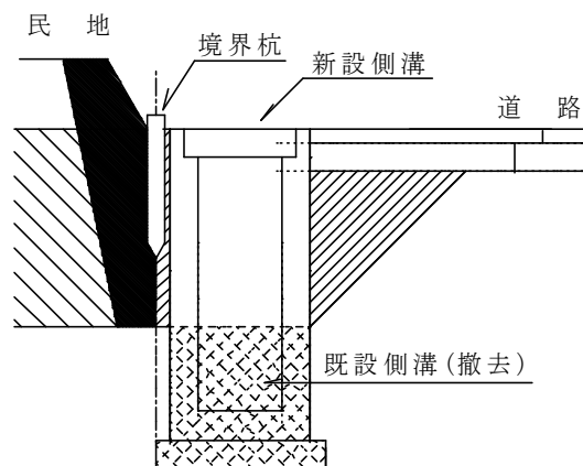
(標準図－４)
