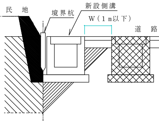
(標準図－２)
