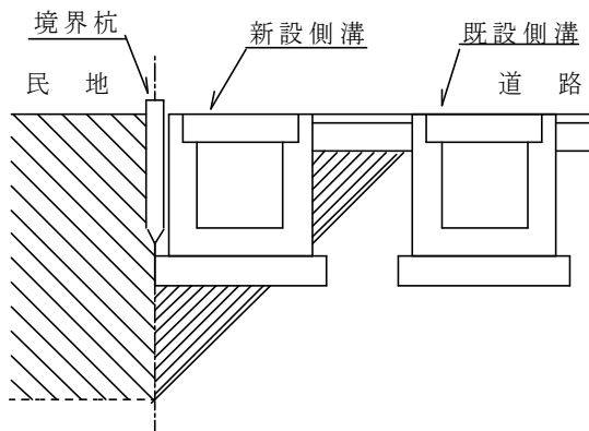
(標準図－１)
