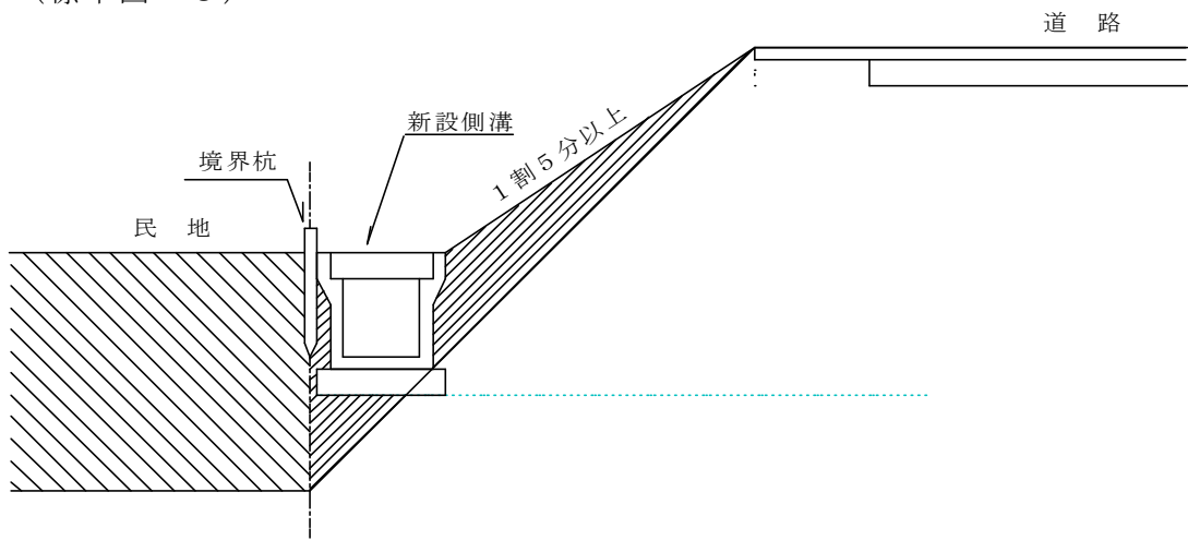
(標準図－３)
