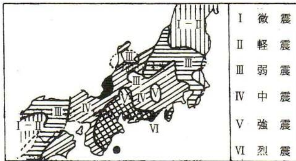
東南海地震の震度分布図
