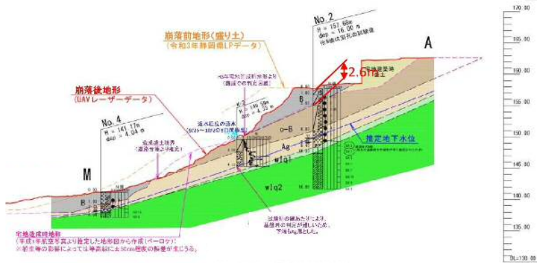
図 地層想定断面図
