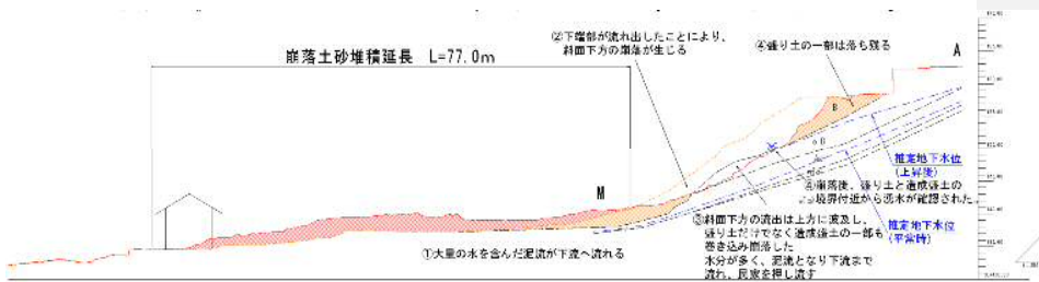
図 崩落後推定断面図
