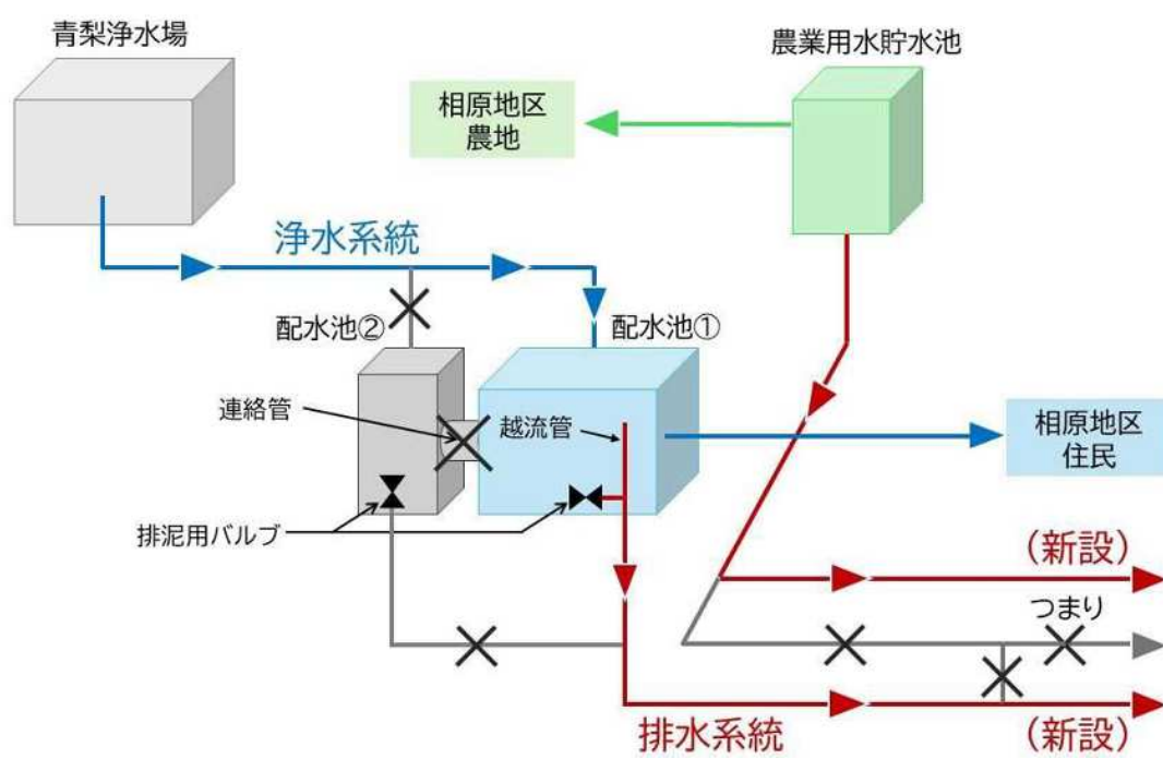
図5 工事後の施設概要図
