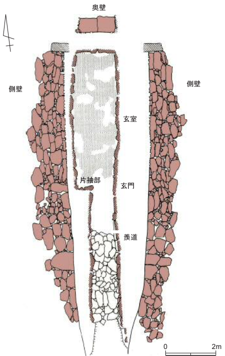
蛭子森古墳 石室実測図
