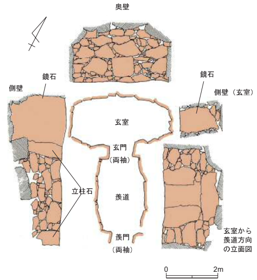
恩塚山古墳 石室実測図
