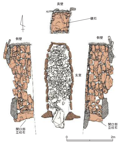
北岡 2 号墳 石室実測図
