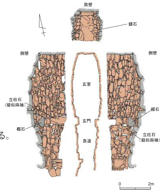
愛宕平古墳 石室実測図
