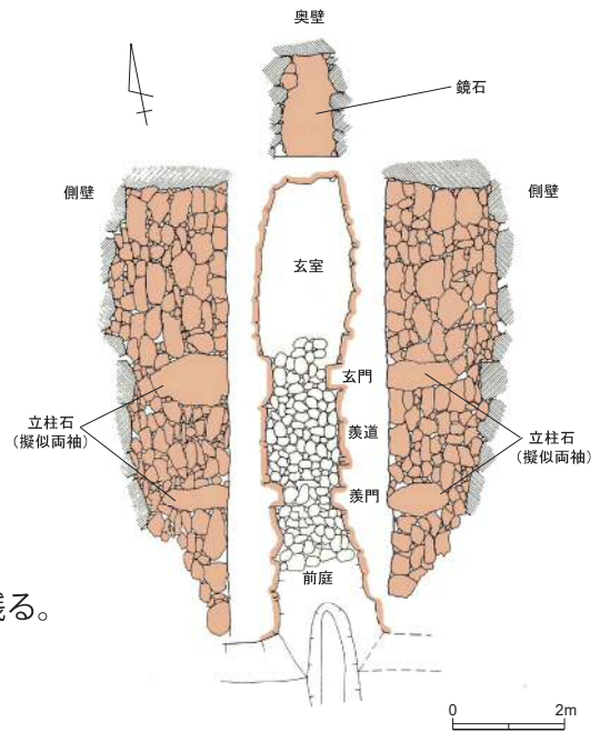
見徳古墳 石室実測図
