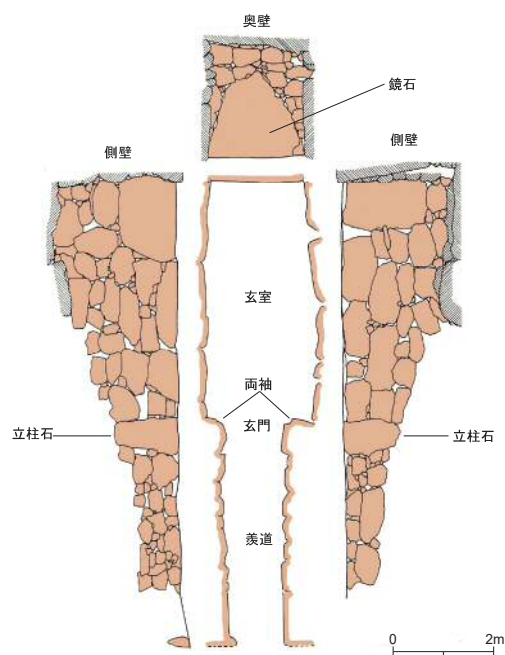
火穴古墳 石室実測図
