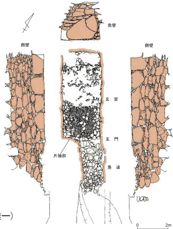
興覚寺後古墳 石室実測図
