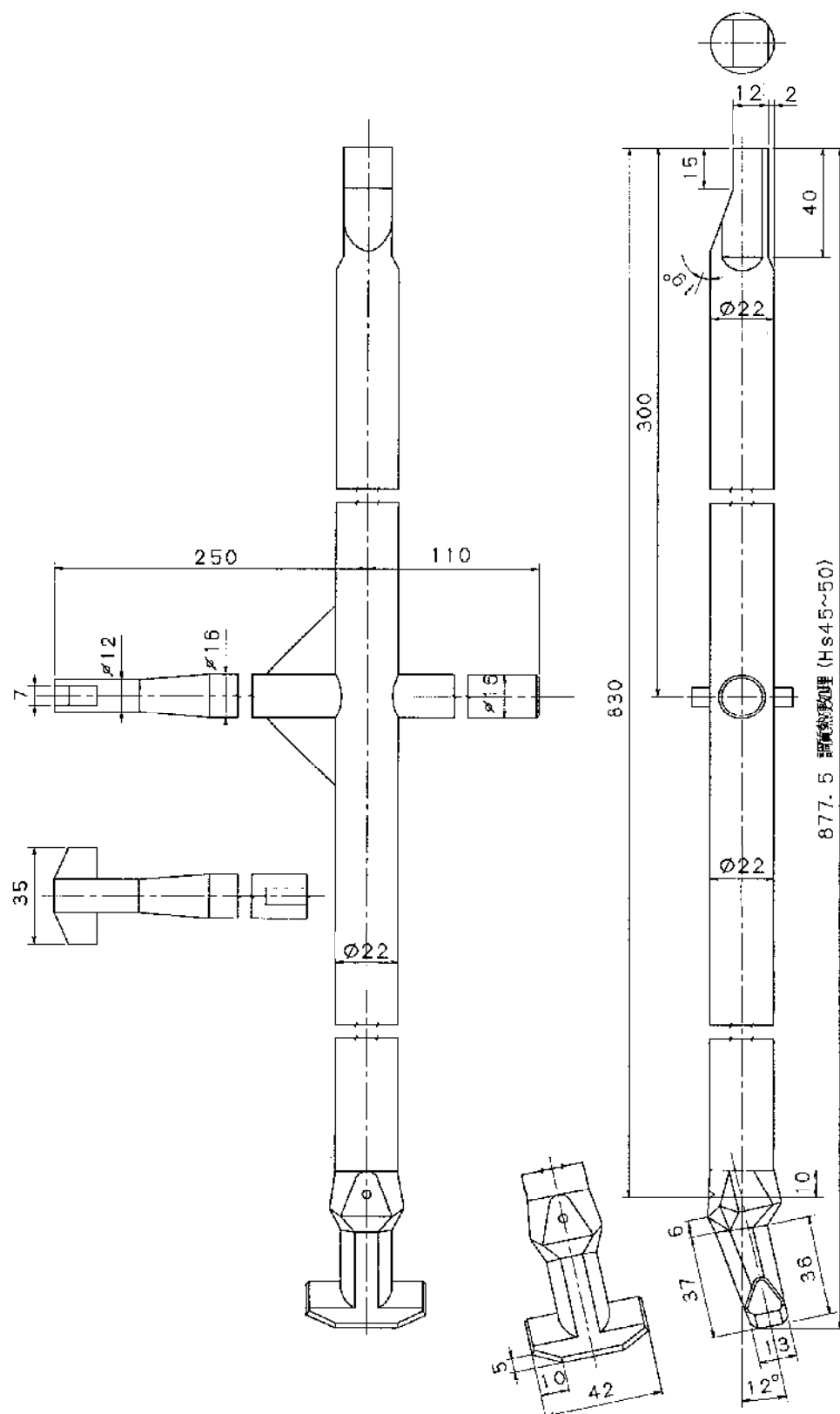
専用工具図
